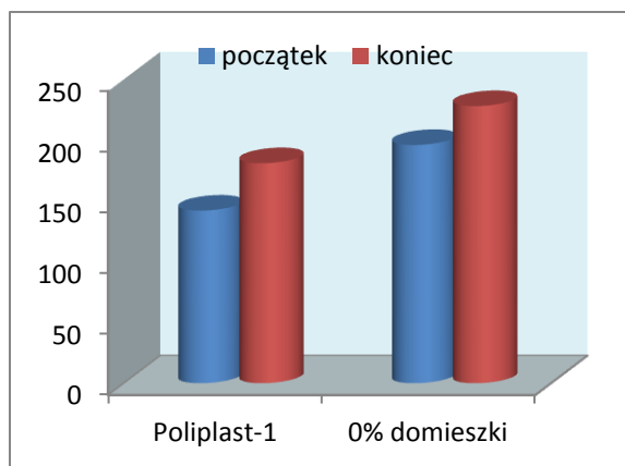
Rys.1. Czas wiązania w temp. 20°C [min]
